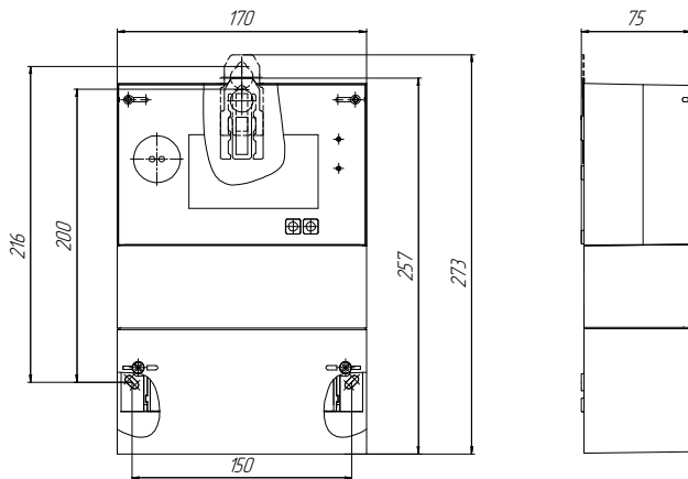
Внешний вид и размеры счётчиков НЕВА СТ4ХХ
