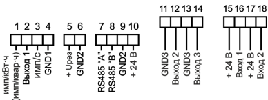
Схема подключения НЕВА СТ4ХХ с дополнительным модулем IO22
